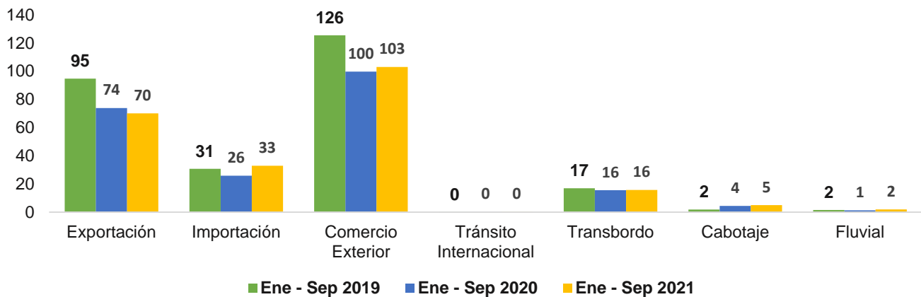
Gráfico 4. Millones de toneladas movilizadas por tráfico portuario de enero a septiembre (2019-2021).
