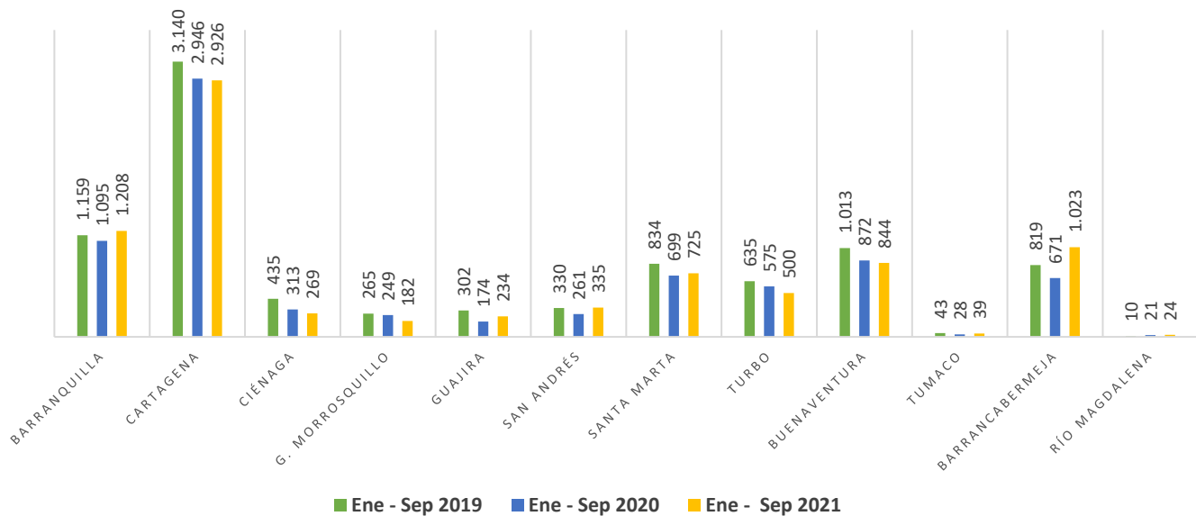
Gráfica 10. Número de arribo de buques por zona portuaria de enero a septiembre (2021).
