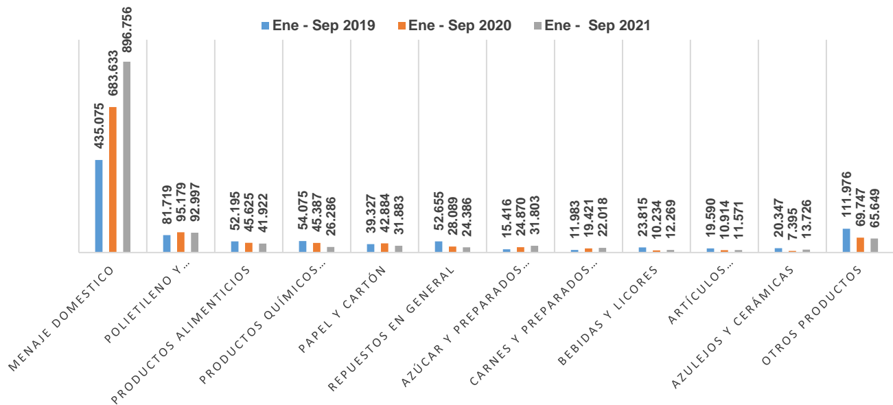
Gráfico 22. Toneladas movilizadas de principales productos importados por SPR Cartagena, enero a septiembre (2019-2021)
