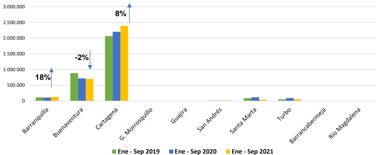
Gráfica 30. Unidades de TEUS por zonas portuarias de enero a septiembre (2019-2021).
