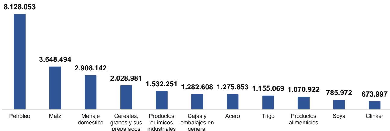
Gráfica 9. Principales productos movilizados por importación de enero a septiembre (2021).
