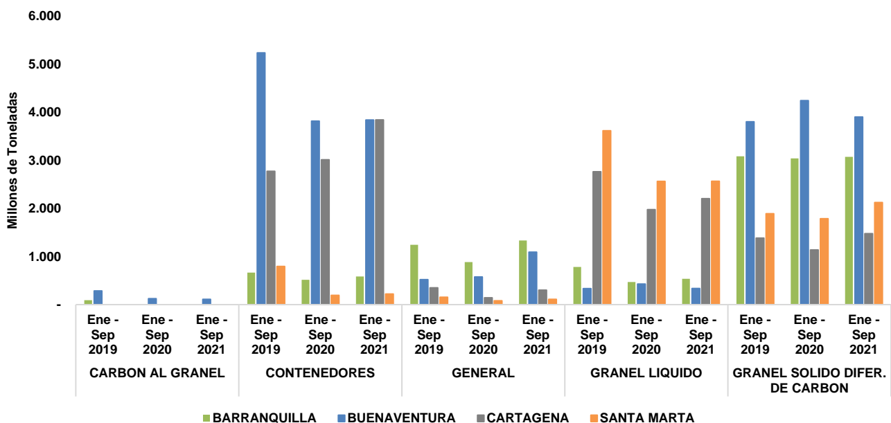
Gráfica 35. Toneladas movilizadas de importación por tipo de carga y zona portuaria (enero a septiembre 2019-2021).
