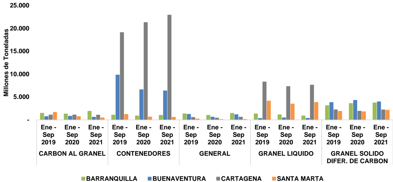
Gráfica 34. Toneladas movilizadas por tipo de carga y zona portuaria (enero a septiembre 2019-2021).
