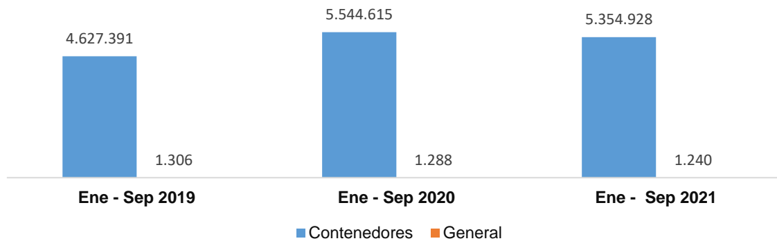
Gráfica 20. Tipo de carga movilizada por la SPR Cartagena de enero a septiembre (2019-2021).
